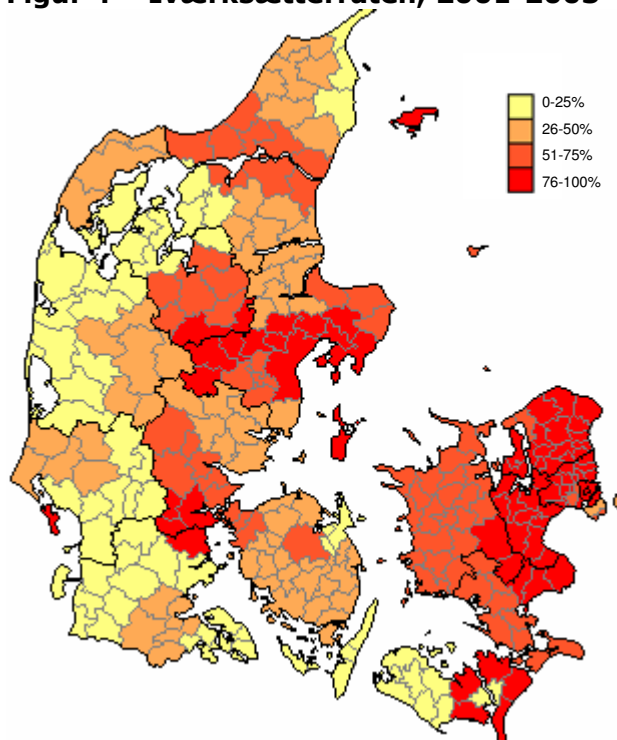
Figur 4 – Iværksætterraten, 2001-2003
